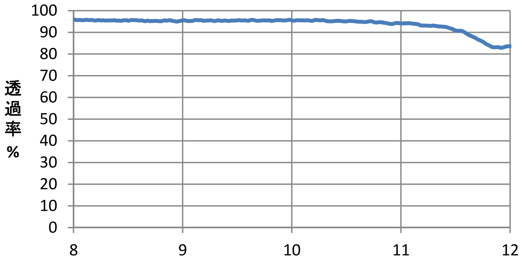
Ge窓8-12um両面AR D30x6t 透過率グラフ(ロット代表)
