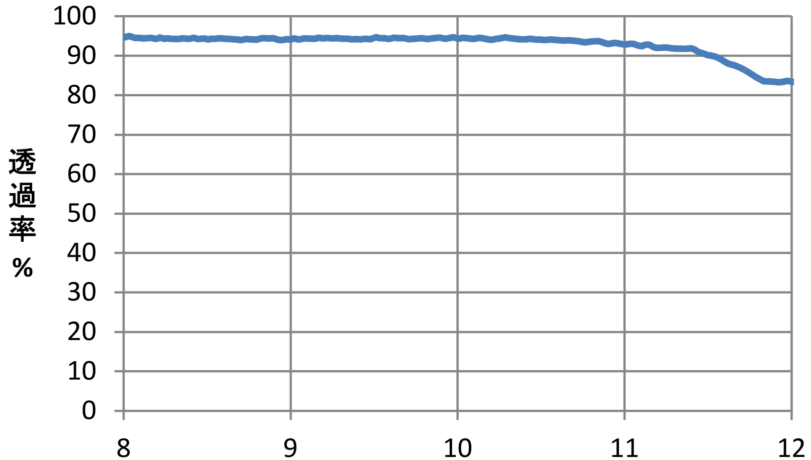
Ge窓8-12um両面AR D30x5t 透過率グラフ(ロット代表)
