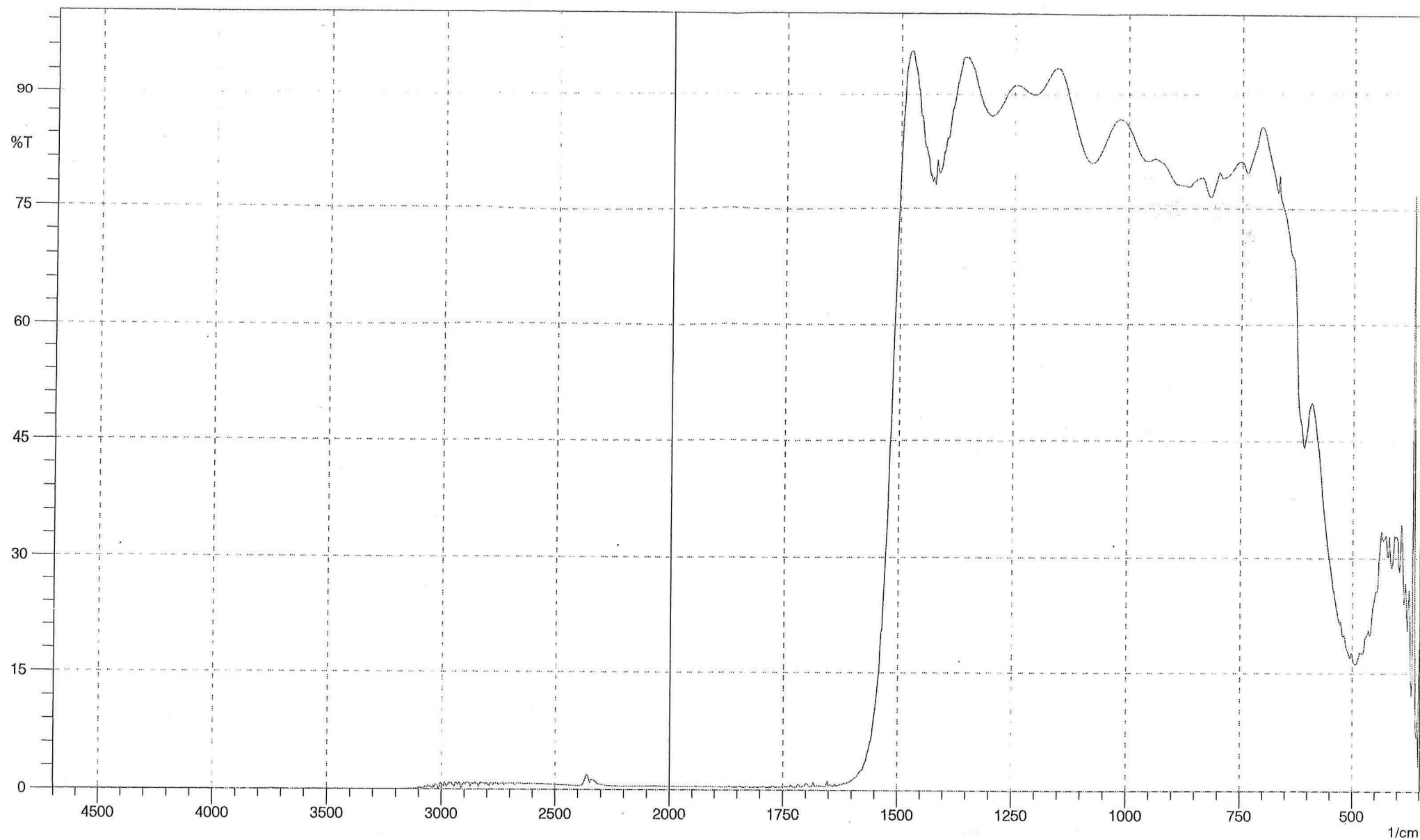
LP-6500 透過率グラフ
