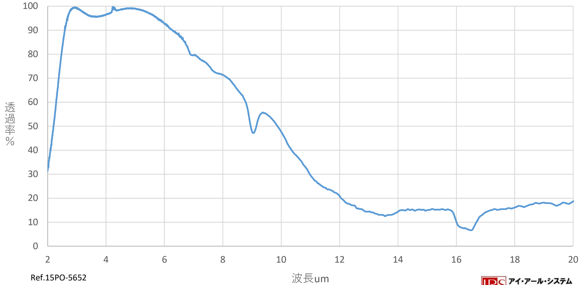
Si窓φ18x1t 3-5umAR/ARコート付 (バッチ代表)
