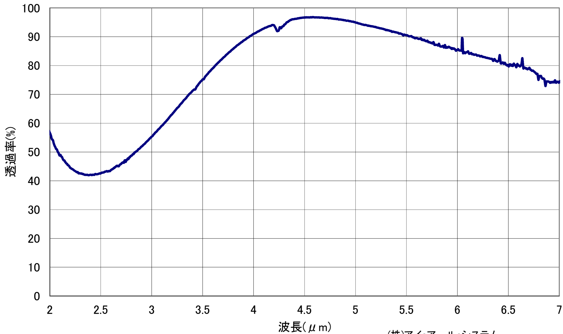
Si(Cz)窓 φ16x1t mm 両面3~5 μm帯ARコート付
