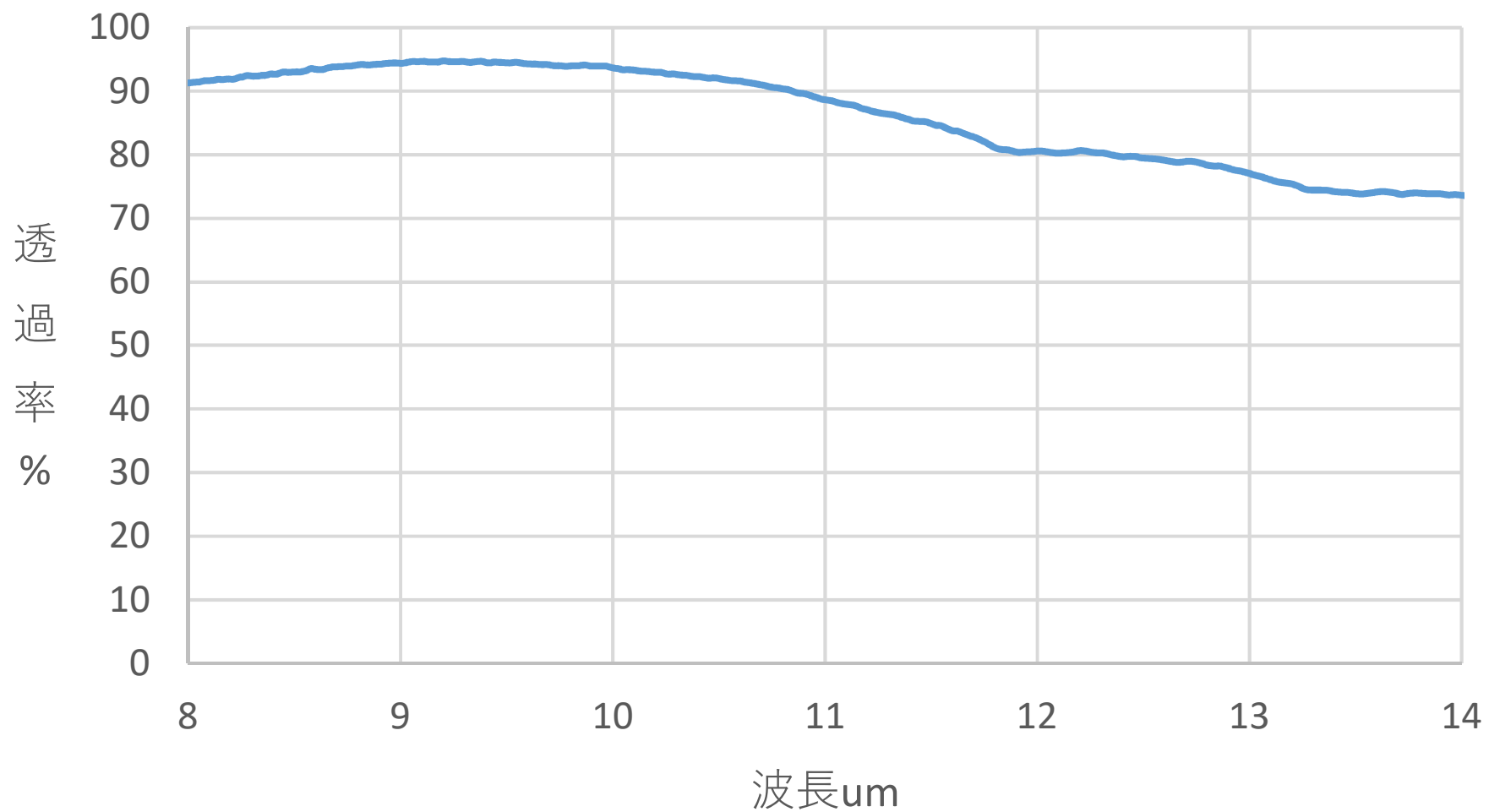
Ge窓D106x3t DLCAR(ロット代表)
