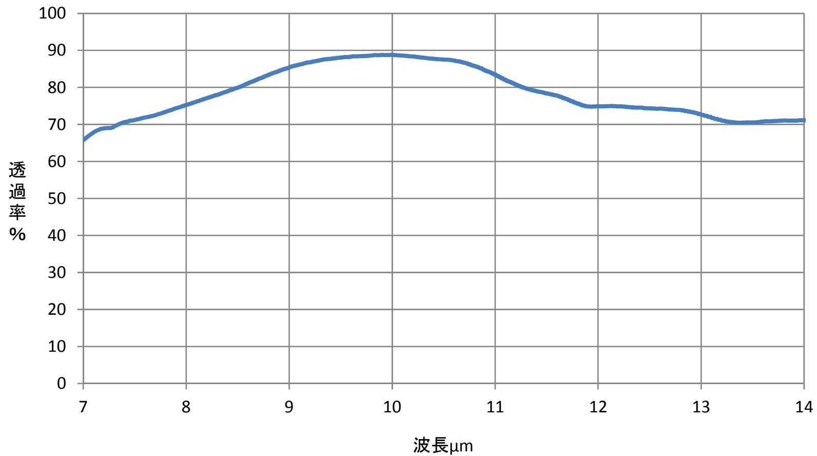
Ge窓8～14μm帯両面DLCコート付 透過率グラフ(ロットサンプル)
