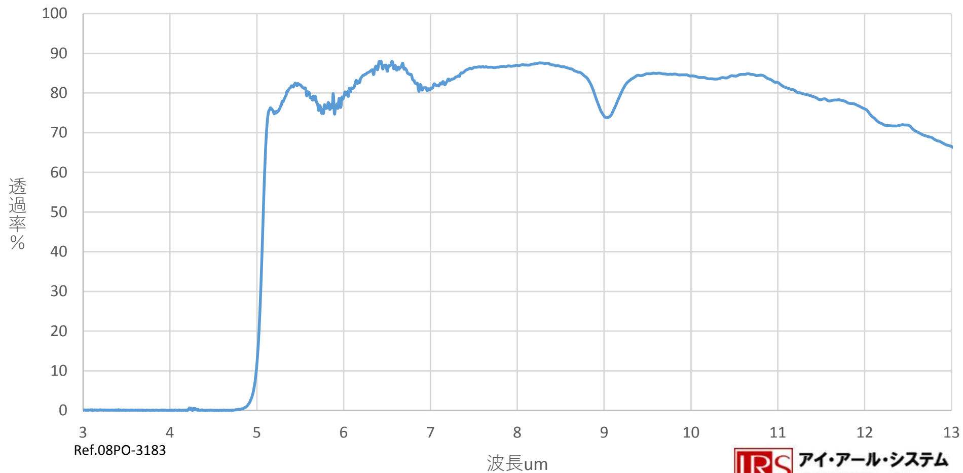
ロングウェーブパスフィルタ LP-5000 \phi 12.5 \times 0.5t (バッチ代表)
