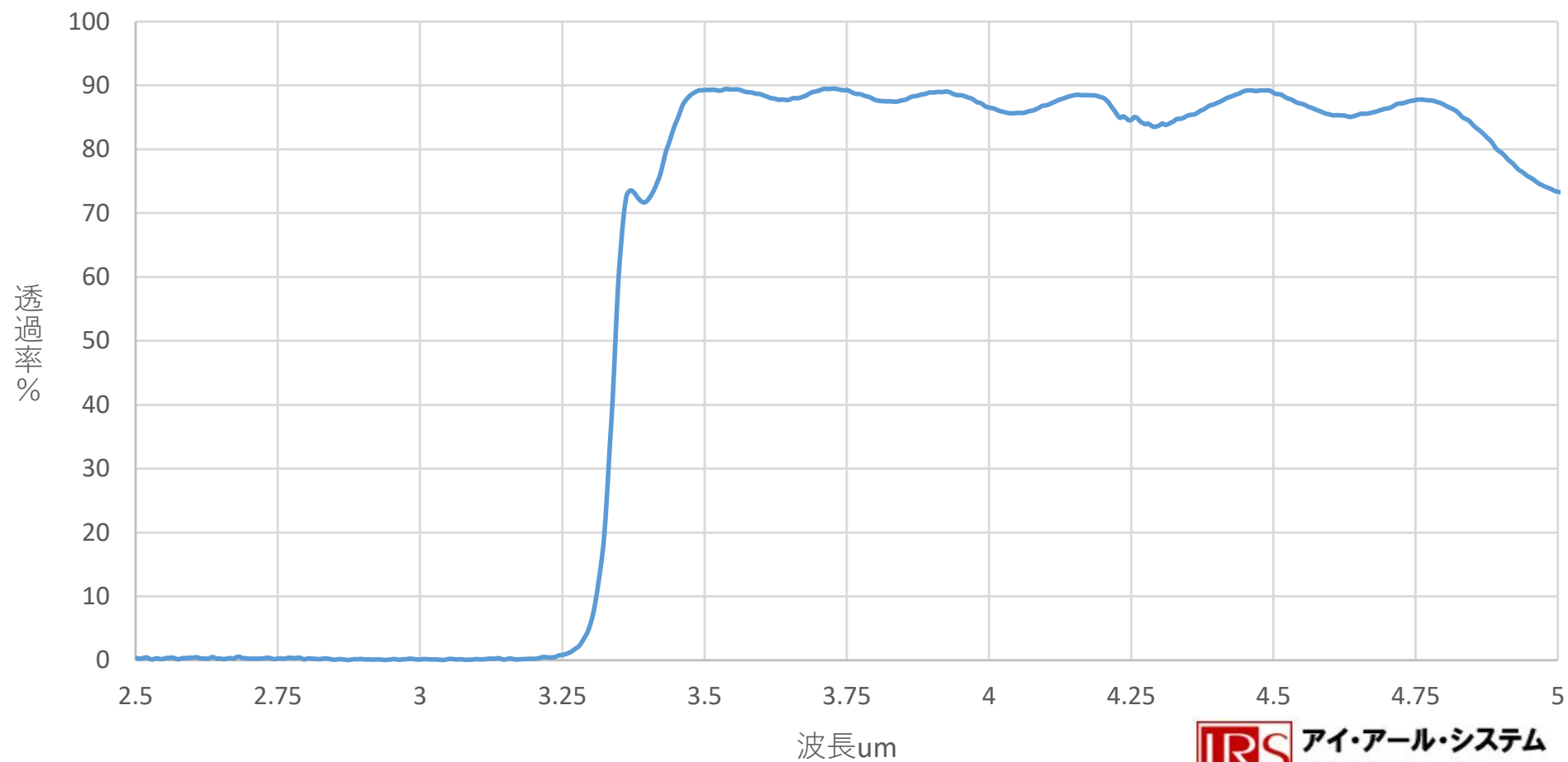
ロングウェーブパスフィルタ LP-3250 D9x1t,0.7c
