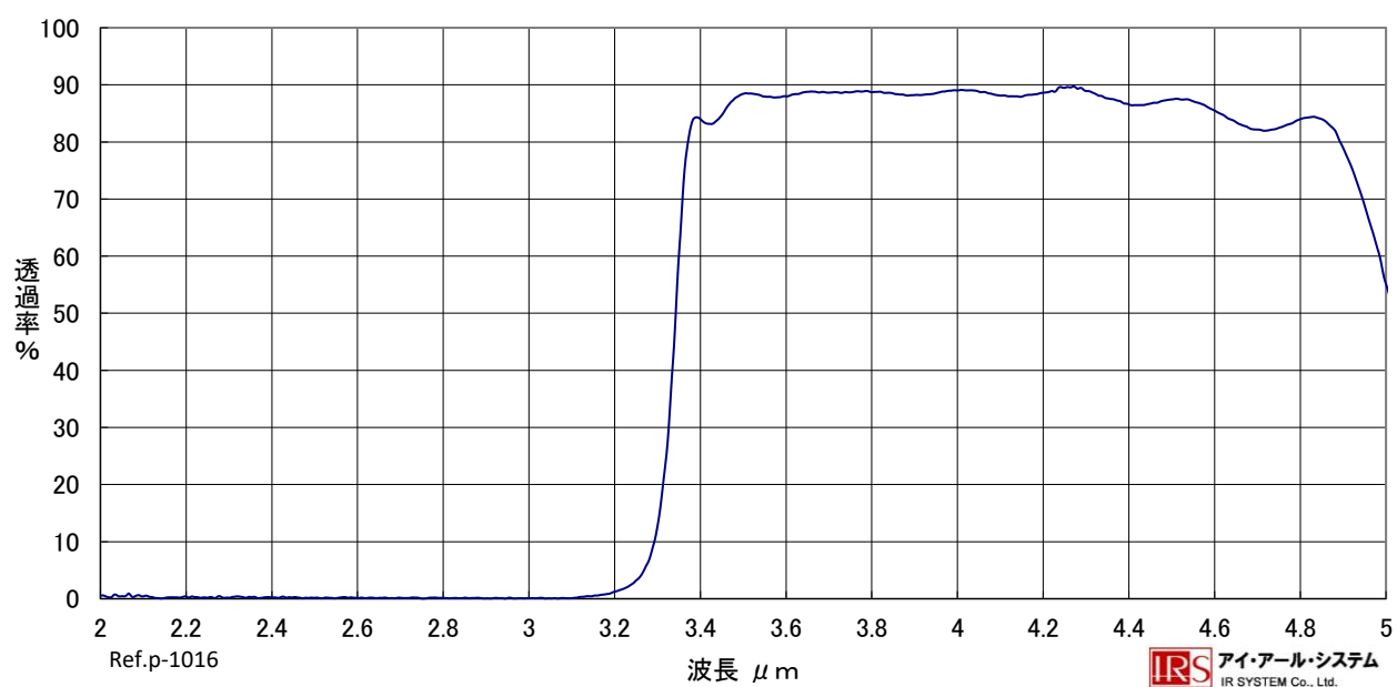
LPF-3250nm D25x1t
