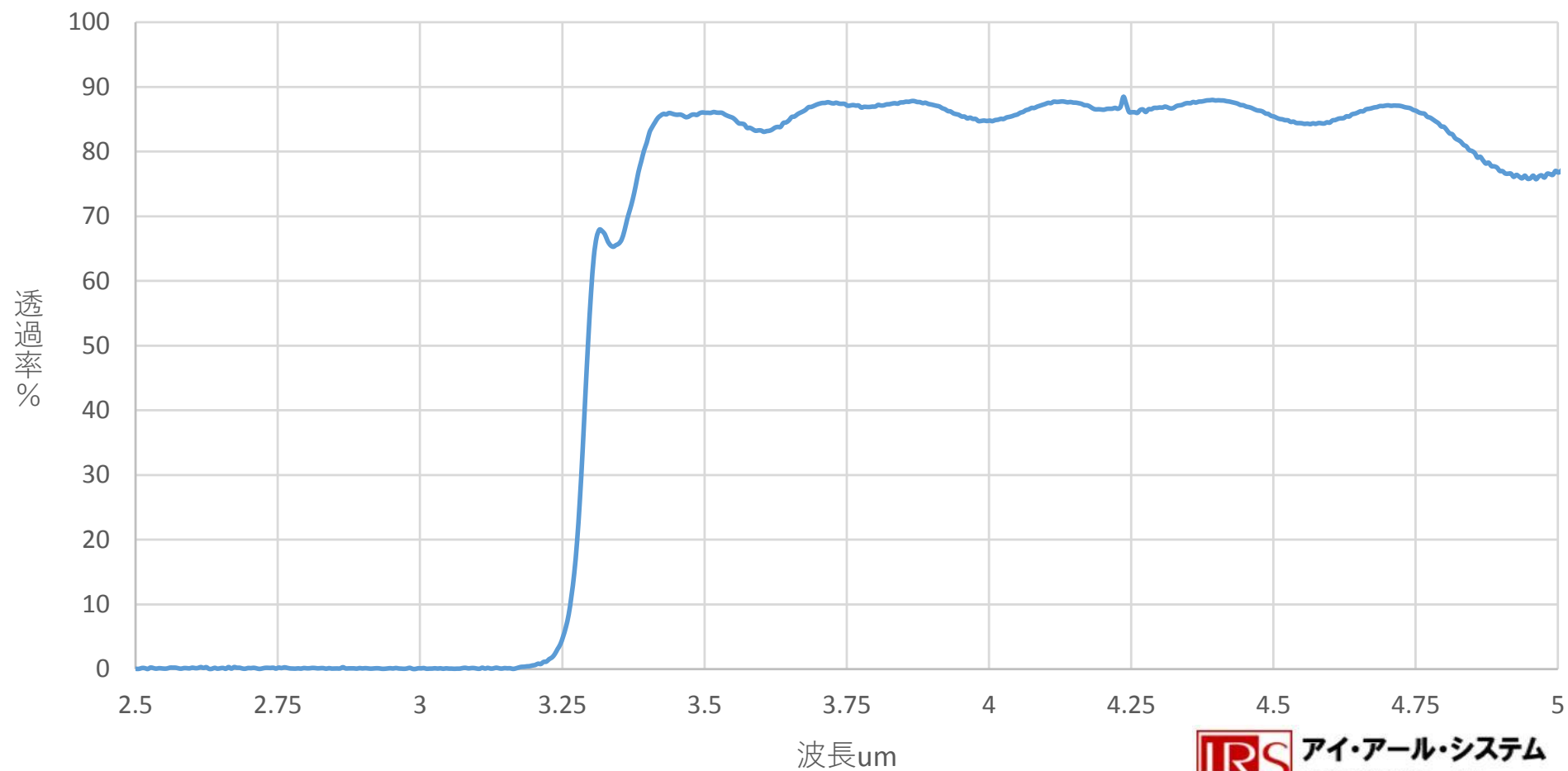
ロングウェーブパスフィルタ LP-3250 \phi 14.5 \times 0.5t 片面コート (バッチ代表)
