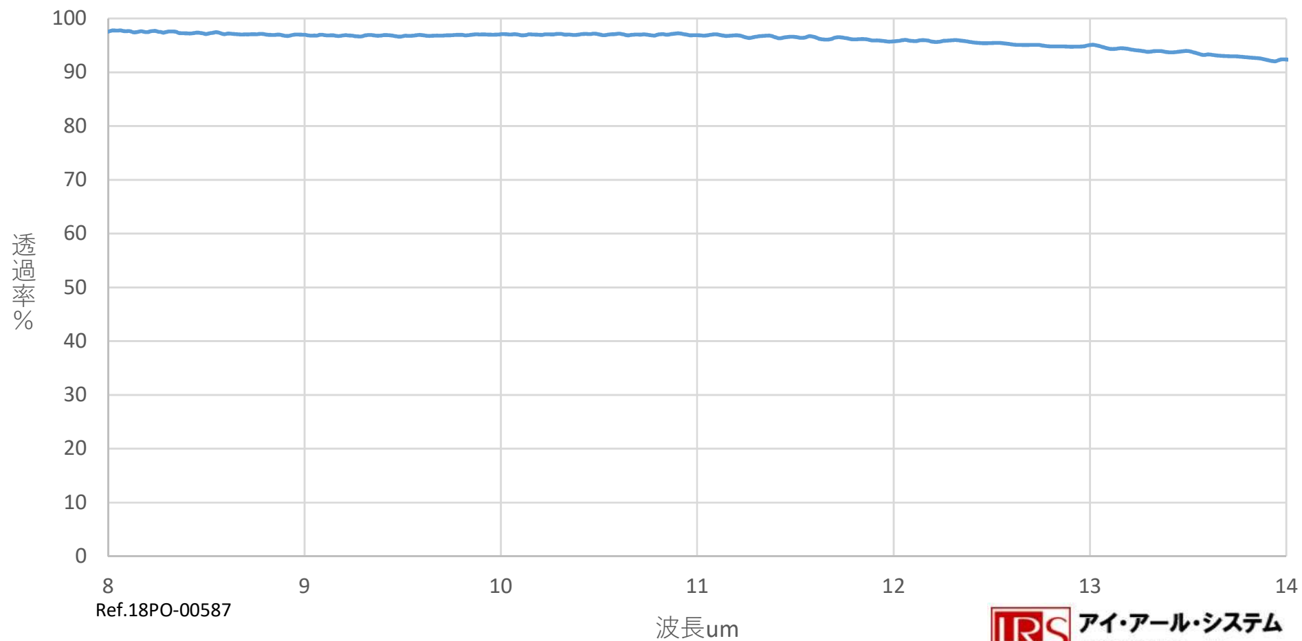
ZnSe窓 D25X1t(mm) 8-14umARARコート付き
