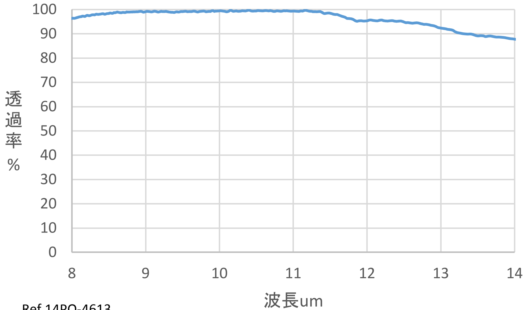
Ge窓D12.5x2t 8-14um両面AR(バッチ代表)
