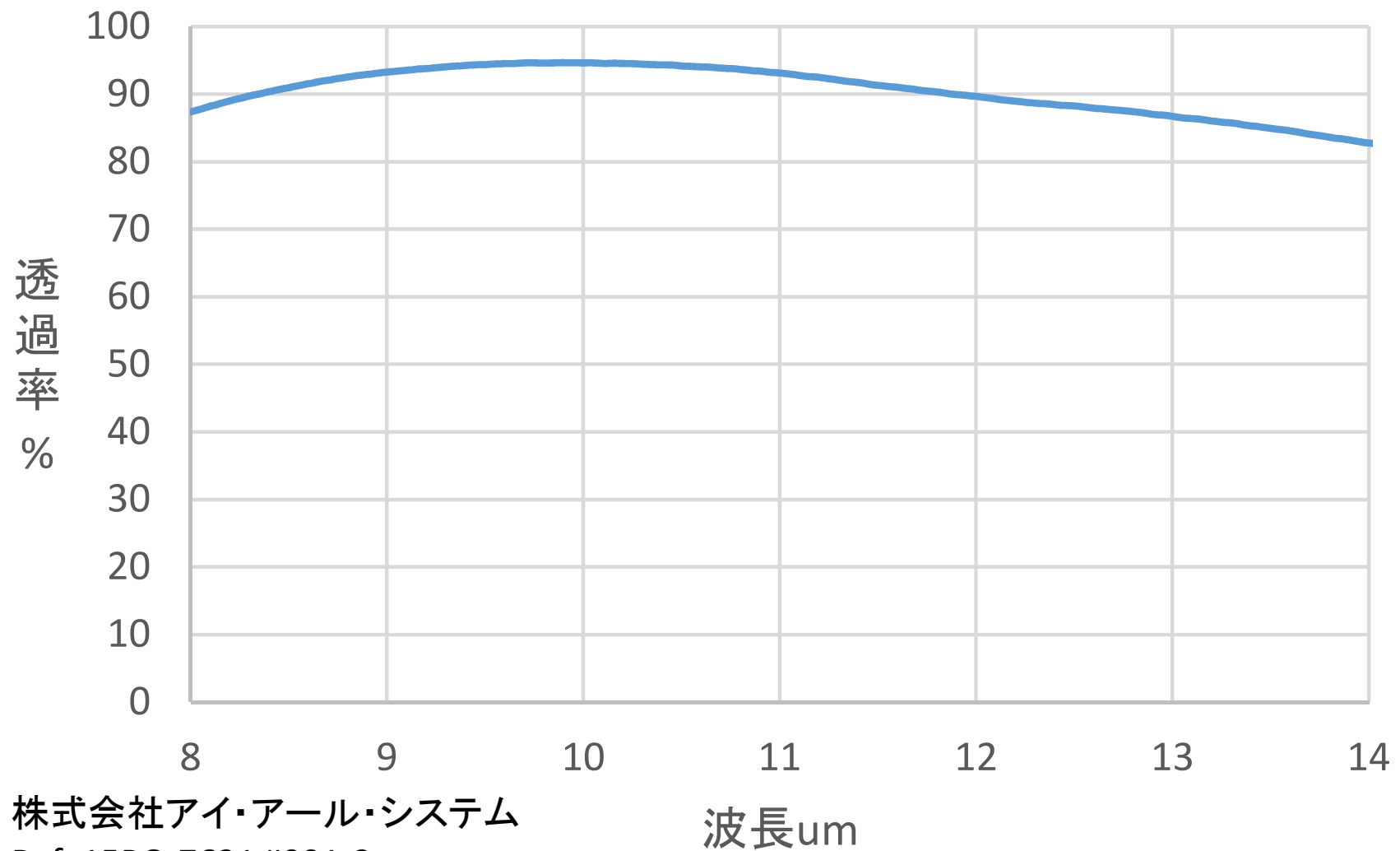
ZnSe窓D60x5t 8-14um両面ARコート 透過率グラフ(代表値)
